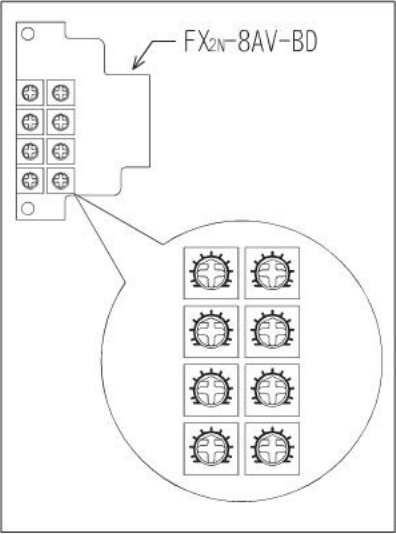
电位器的放大图
