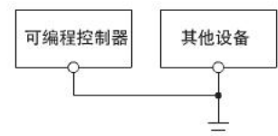
共同接地 (不允许)
