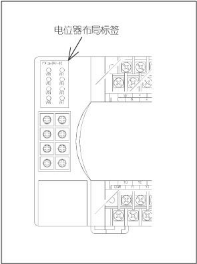
标签粘贴的范例
