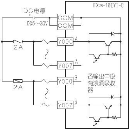
接线示例
