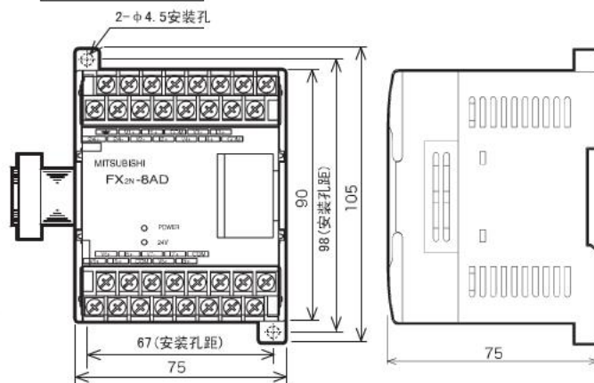
FX2N-8AD 重量: 0.4kg
