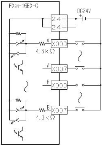
接线示例
