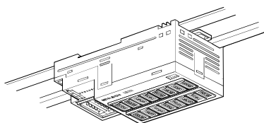
図 2.4 天井取付け Fig. 2.4 Ceiling installation
