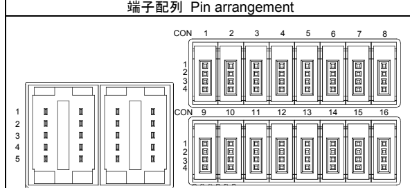
ユニットの正面から見た場合 A module view from the top
