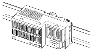
図 2.2 正面取付け (逆方向) Fig. 2.2 Front installation (Upside-down orientation)
