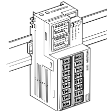
図 2.3 正面取付け (縦方向) Fig. 2.3 Front installation (Vertical orientation)
