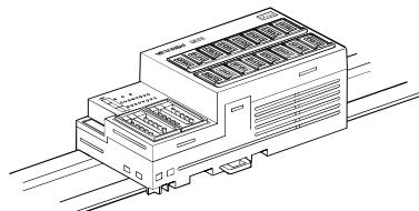
図 2.5 平面取付け Fig. 2.5 Horizontal installation
