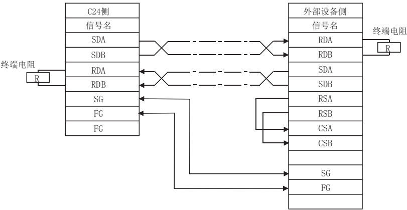
(b) 外部设备与 C24 以 1: n(多点)方式连接的情况下
