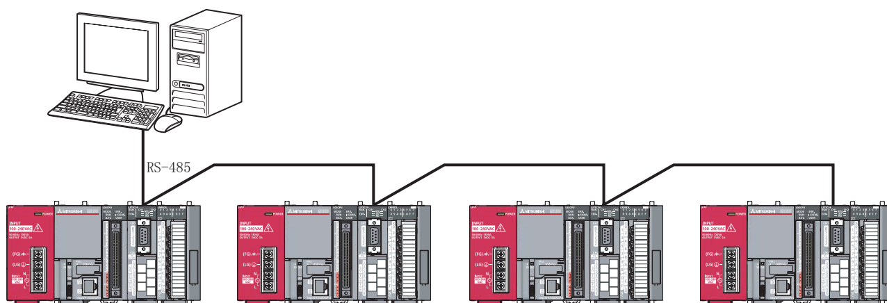
(c) 外部设备与 C24 采用 1: n 的系统配置的情况
