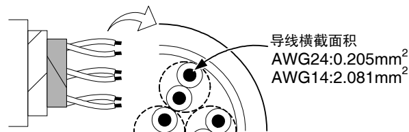
电缆参考图
