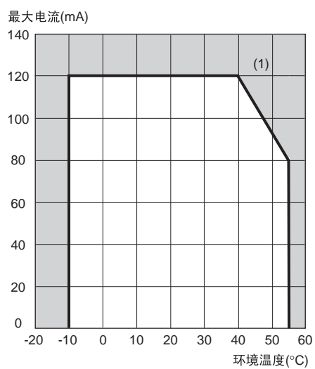
12 V 电源
