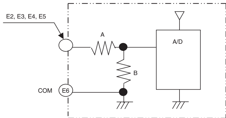
电路图
