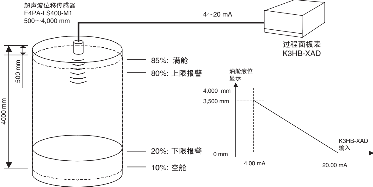
接线图
