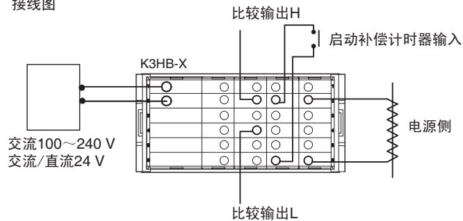
接线图
