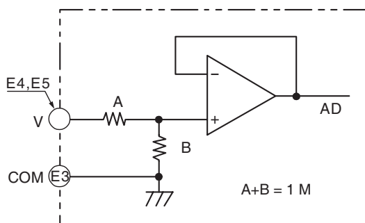
电路图
