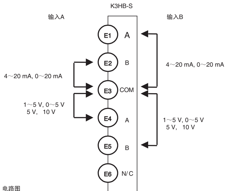
电路图
