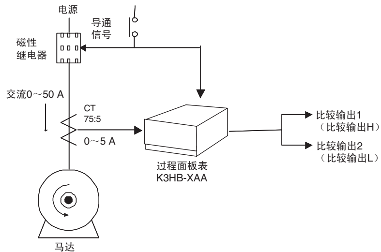
接线图
