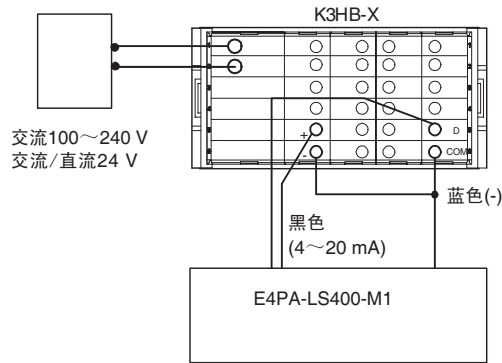
接线图
