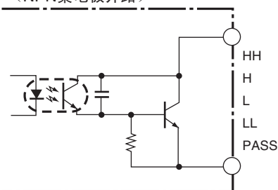
晶体管输出时 (NPN集电极开路)
